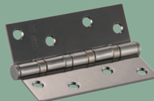
100×70×2.5 4BB BLACK NICKEL Чёрный никель
